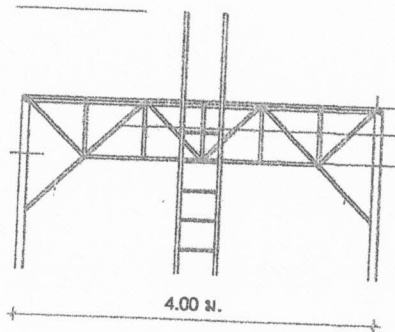
แบบขยายโครงเหล็กรับถังน้ำ มาตราส่วน 1 : 50
