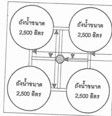
แบบขยายการเชื่อมต่อถังน้ำขนาด 2,500 ลิตร
