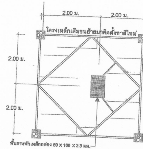
แปลนชั้นที่ 2, 3 ขนาดหน้า 1 : 50
