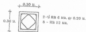
ขยายเสา
