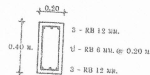
ขยายคาน GB
