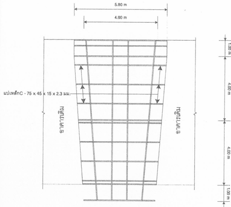
แปลนโครงหลังคาเมทัลชีท 1 : 100
