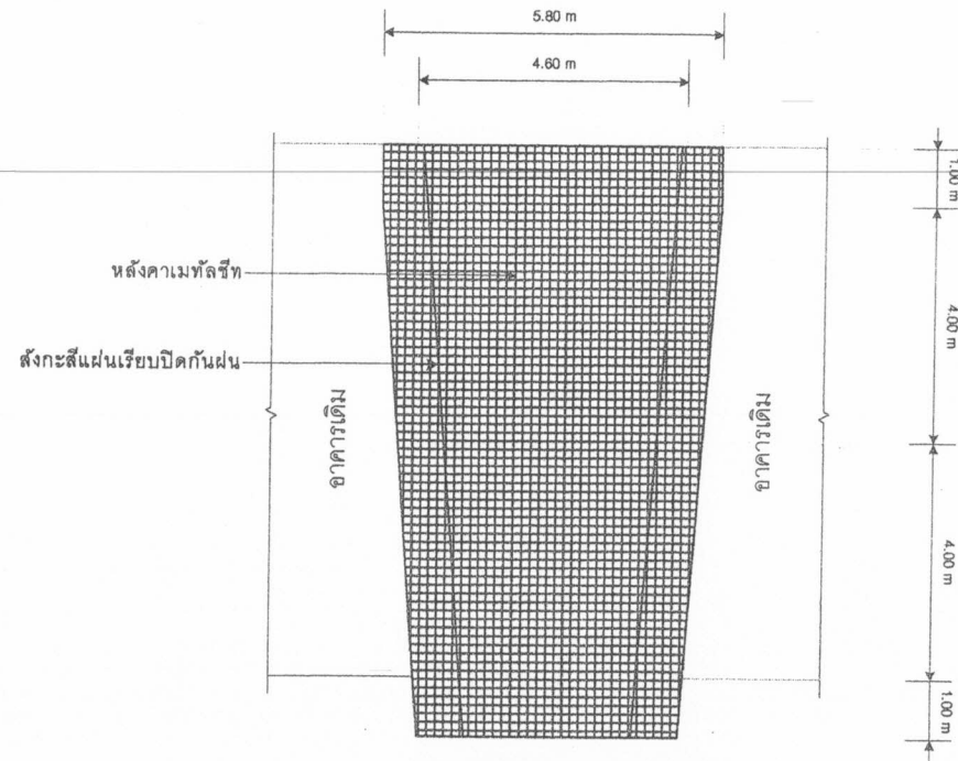
แปลนหลังคาเมทัลชีท 1 : 100
