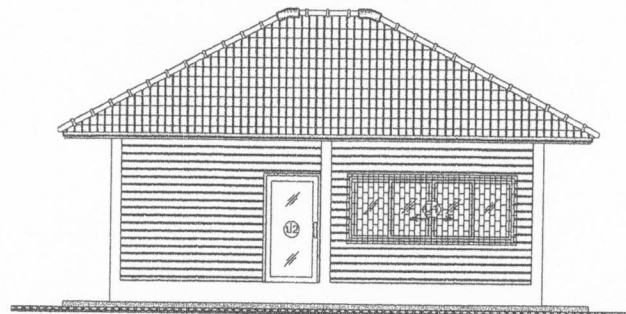
รูปด้านซ้าย 1 : 100
