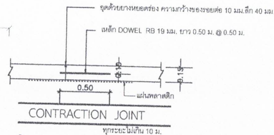
รูปตัดถนน
