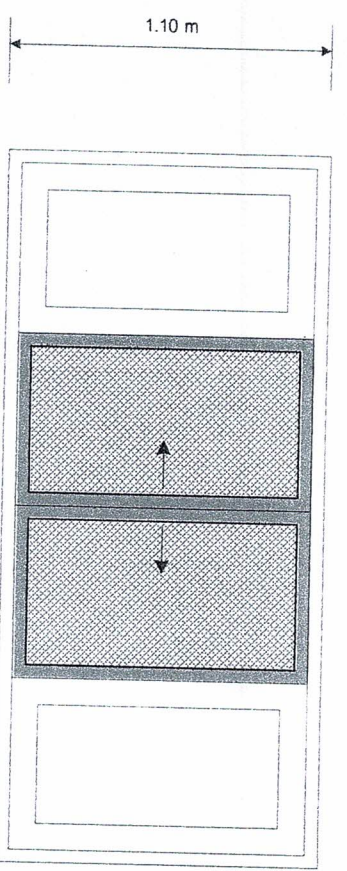
บานมุ้งลวดหน้าต่าง ขนาด 1.10 X 2.60 ม.
