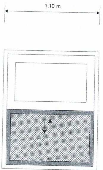
บานมุ้งลวดหน้าต่าง ขนาด 1.10 X 1.50 ม.
