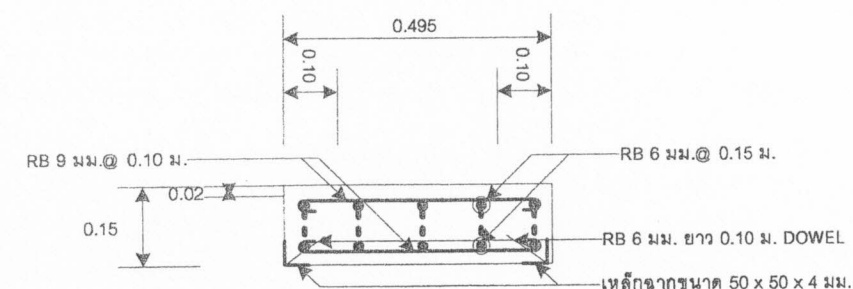
รูปตัดฝารางระบายน้ำ ค.ส.ล. 1 : 10
