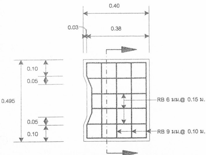
รูปฝารางระบายน้ำ ค.ส.ล. 1 : 10
